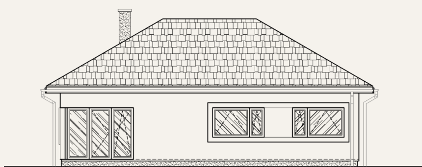
ELEWACJA TYLNA
