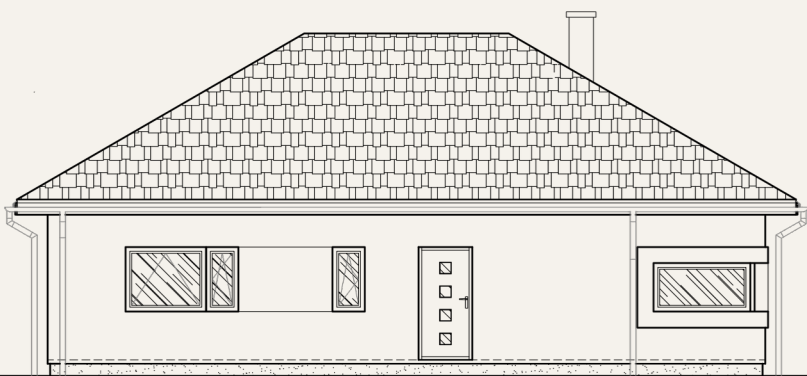
ELEWACJA FRONTOWA
