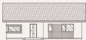
ELEWACJA FRONTOWA
