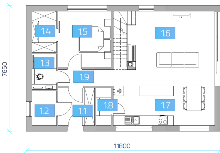
RZUT PARTERU
