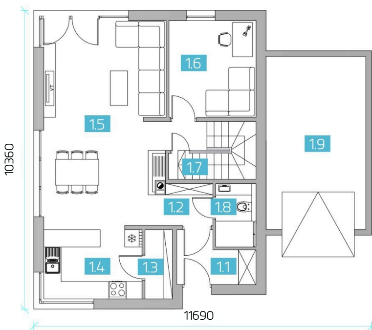
RZUT PARTERU
