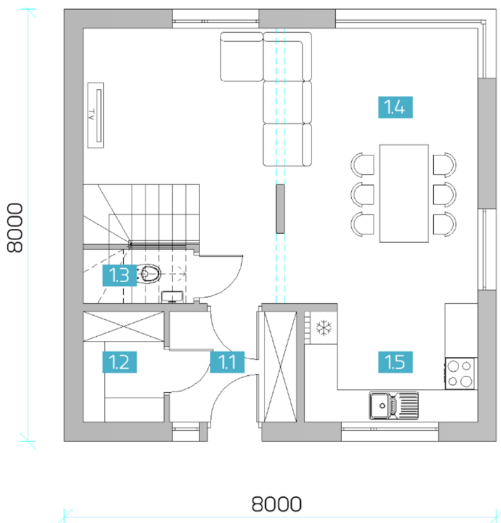
RZUT PARTERU
