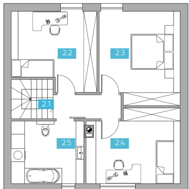
RZUT PODDASZA
