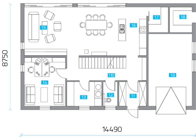
RZUT PARTERU
