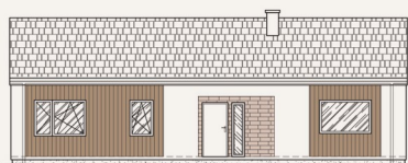
ELEWACJA FRONTOWA
