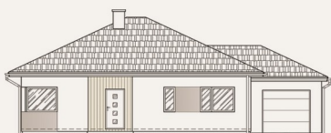
ELEWACJA FRONTOWA
