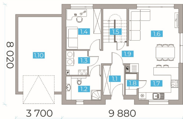
RZUT PARTERU
