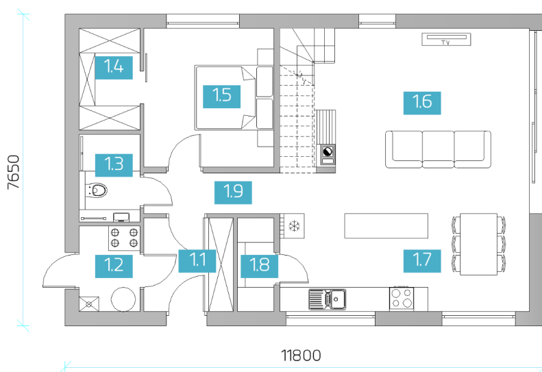
RZUT PARTERU
