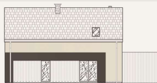
ELEWACJA TYLNA
