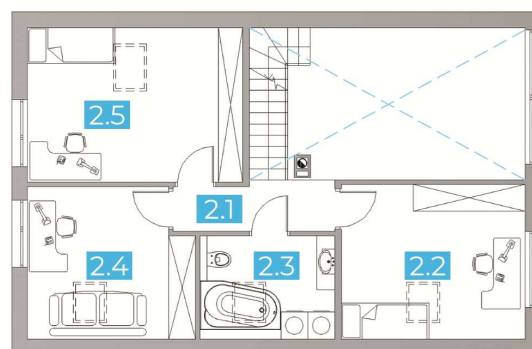
RZUT PODDASZA
